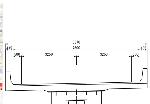
標準横断面図
