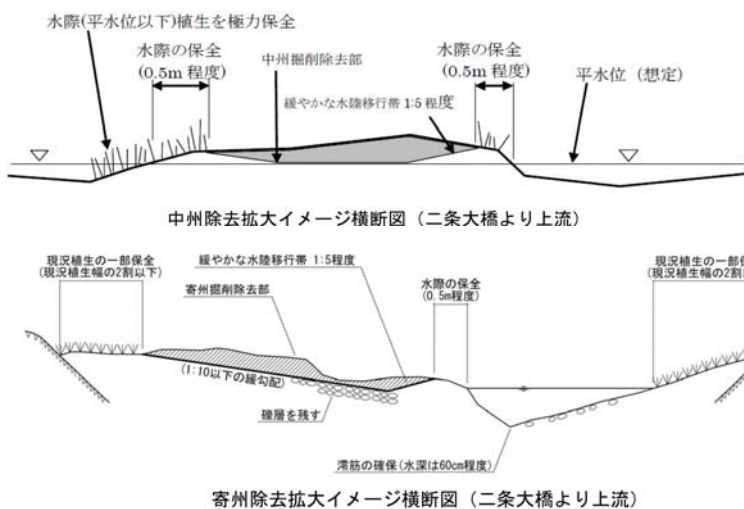
実施イメージ横断面図
