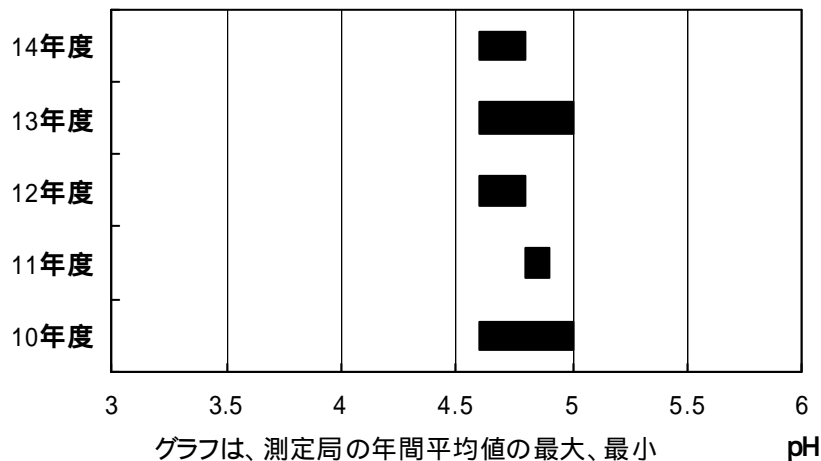
図3-4 府内降水のpH値(平均値)の経年変化
