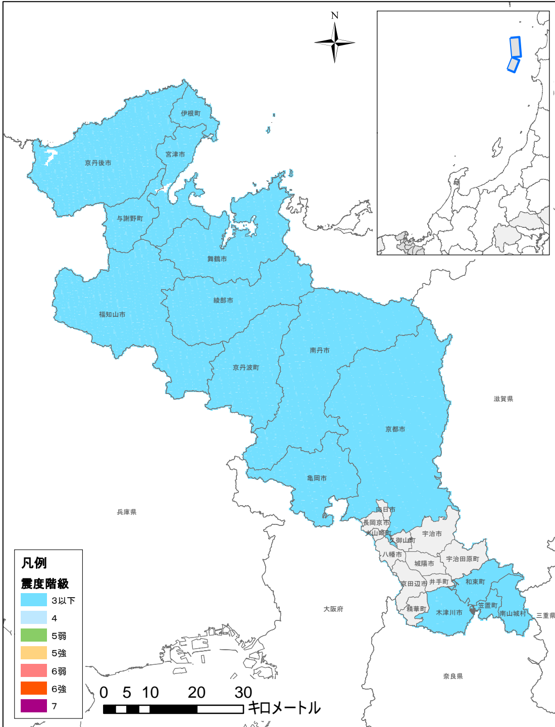
図 2(1)② 震度分布図 (相田 1984) (グリーン関数+距離減衰)
