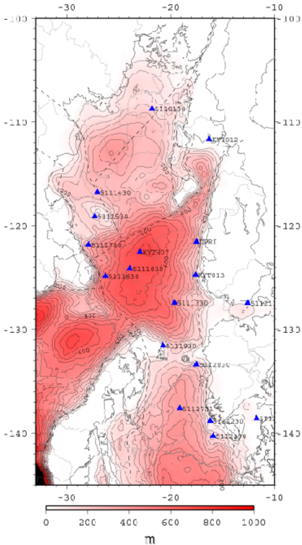
図-4 重力による基盤岩深度分布と地震観測点
