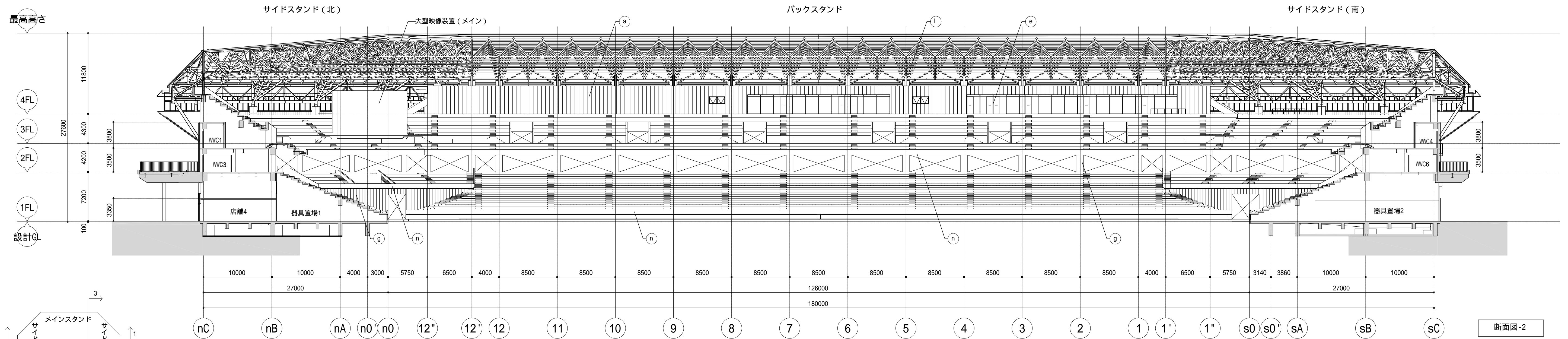
断面図-1
