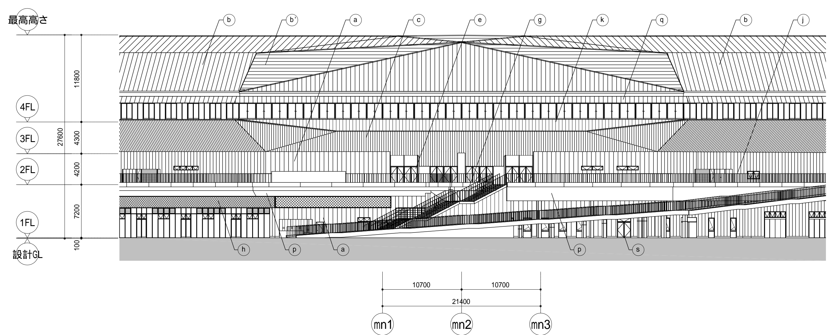
北西立面図
