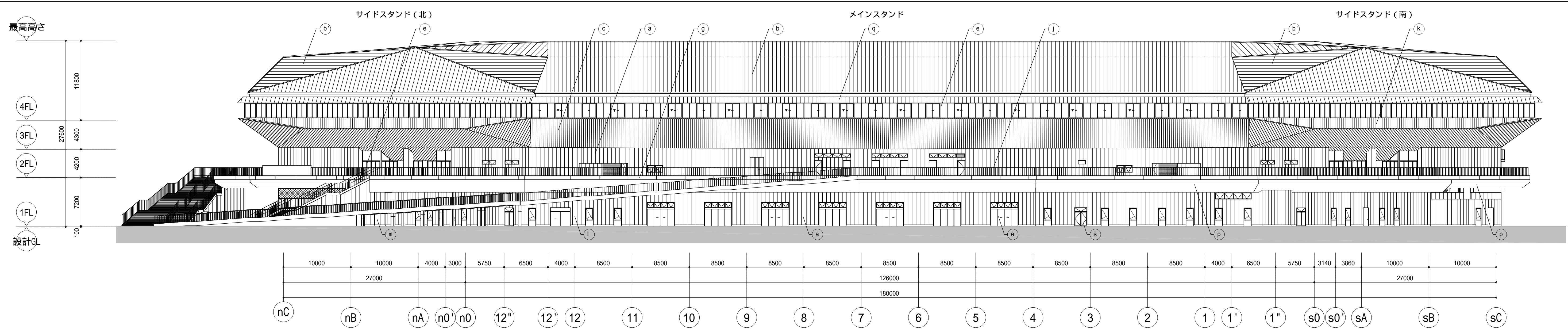
西立面図
