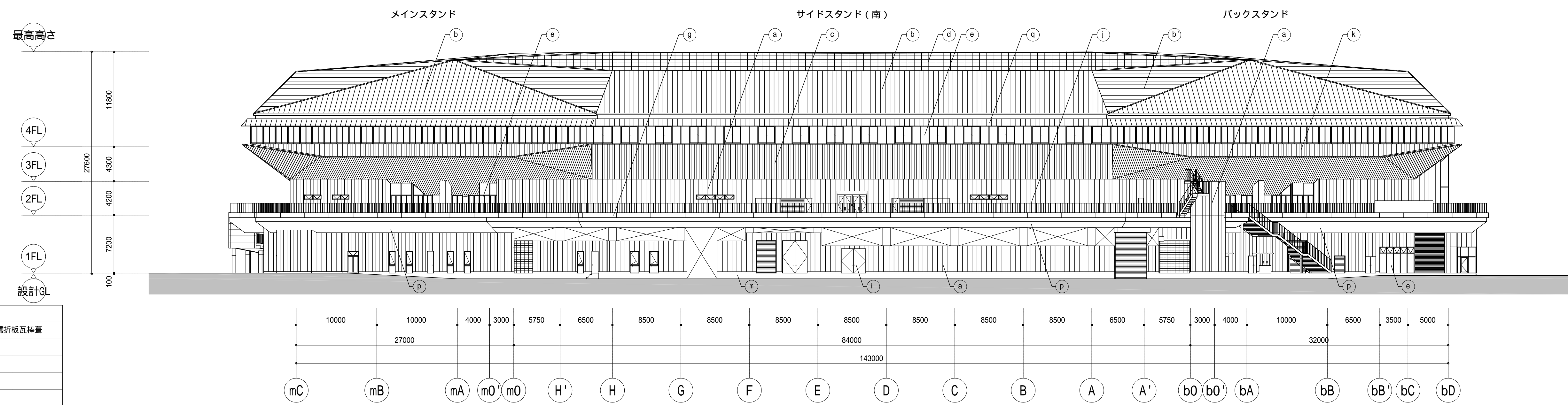
南立面図
