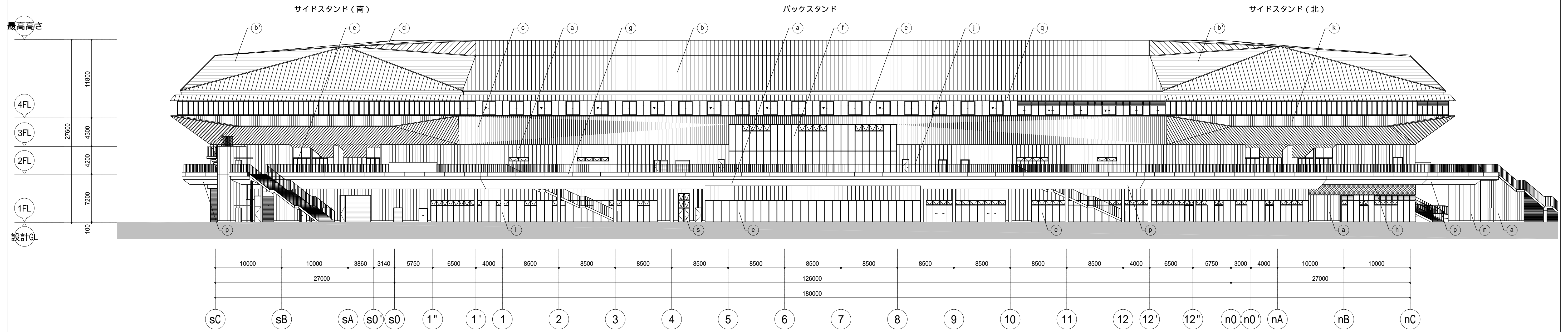
東立面図
