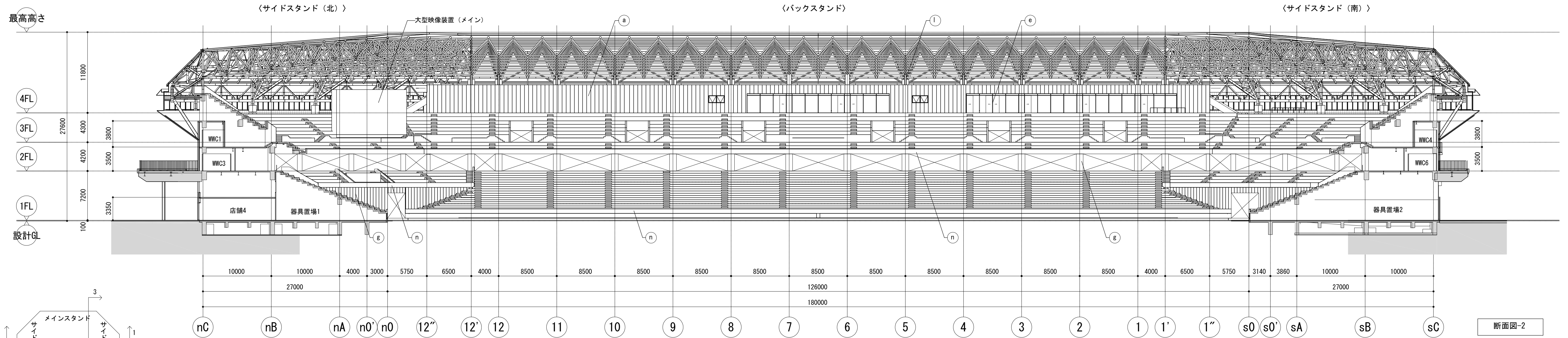
断面図-1
