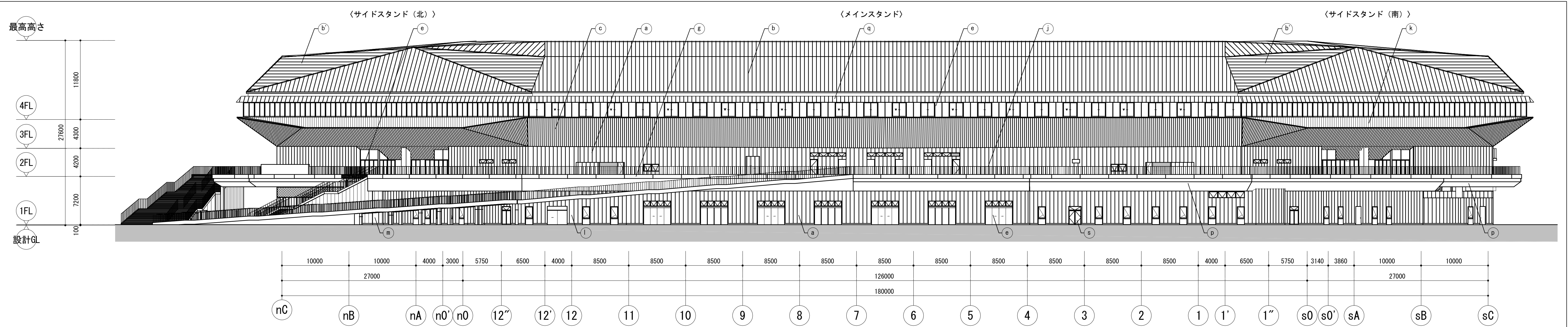
西立面図
