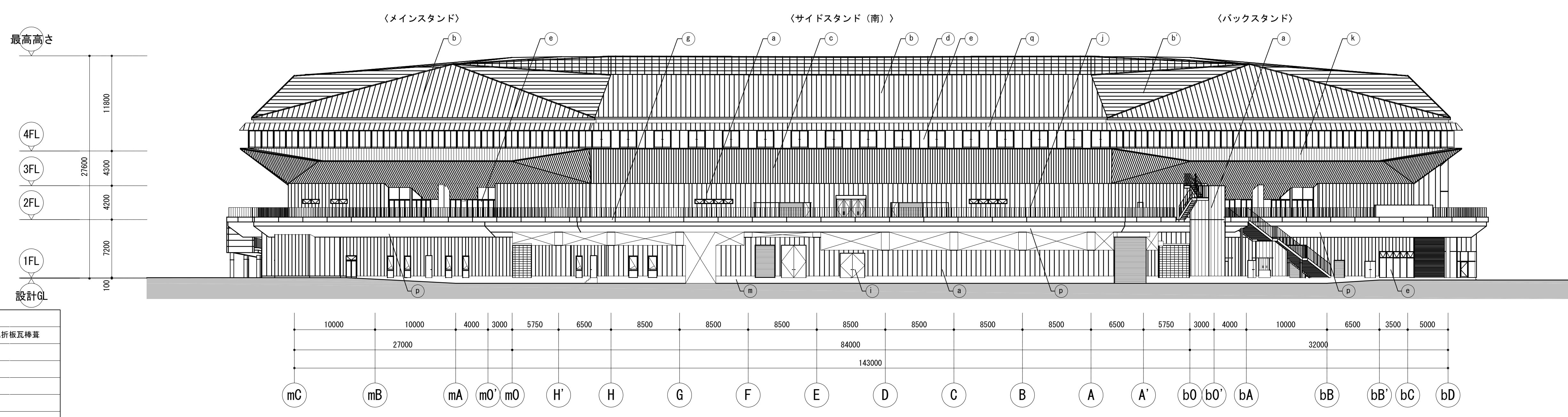
南立面図
