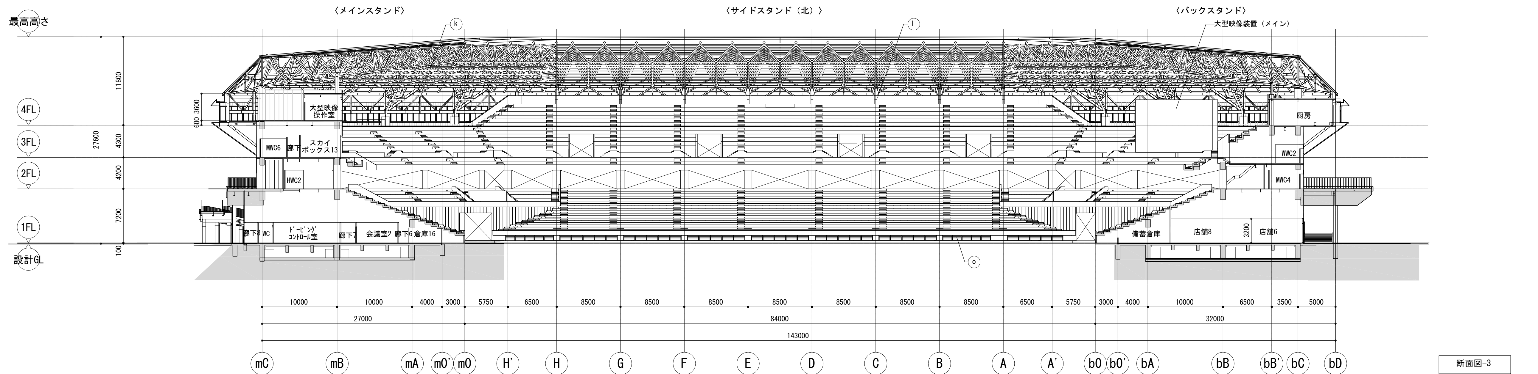
断面図-2
