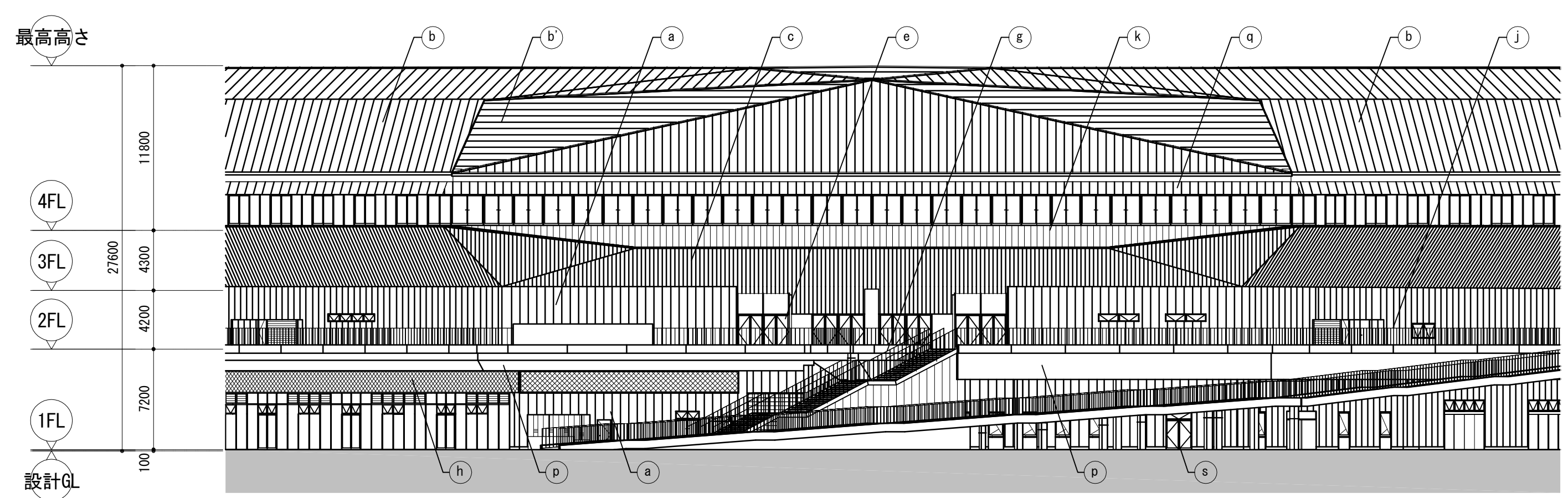
北西立面図
