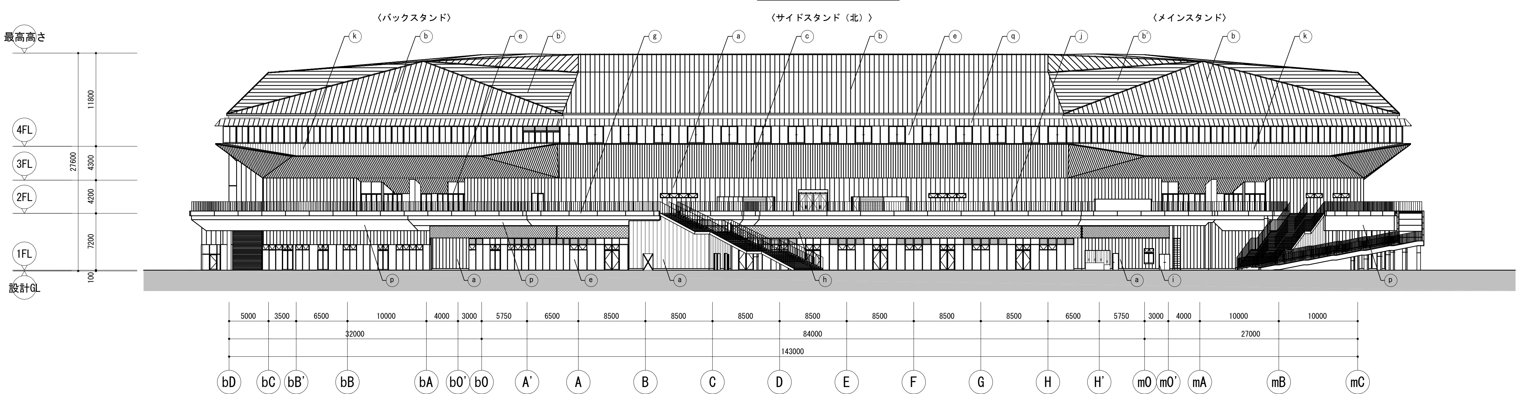
北立面図
