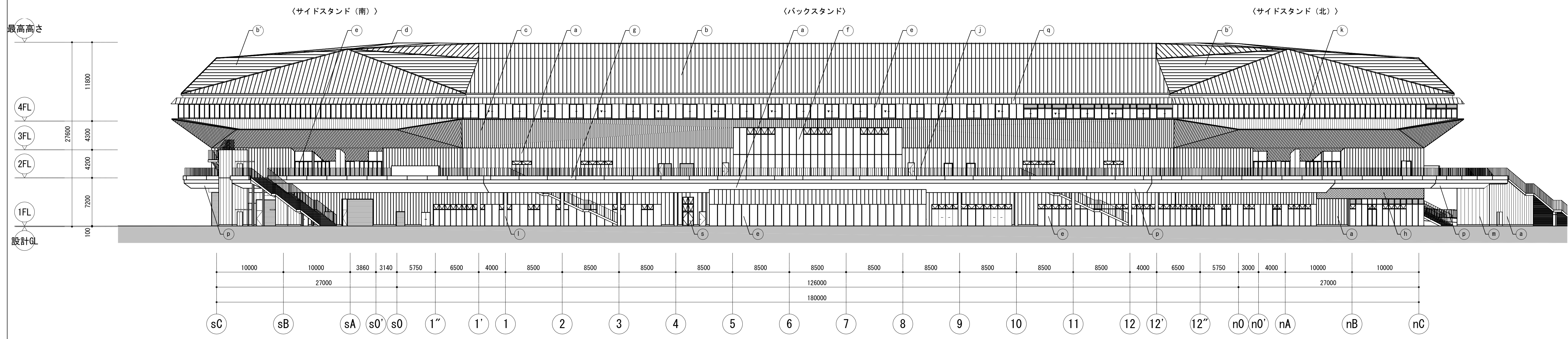
東立面図
