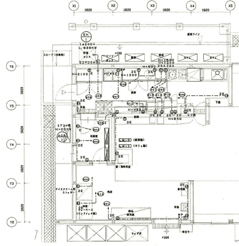
平面図 1/50 コミュニケーション配線
