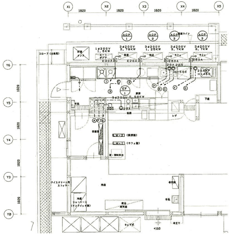
平面図 1/50 動力配線
