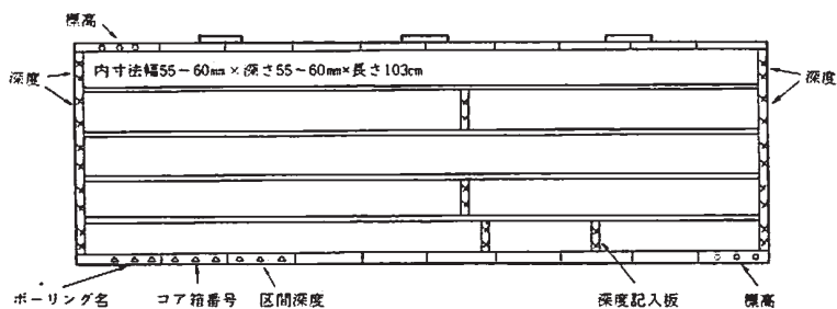
図 4. 1 コア箱記入例
