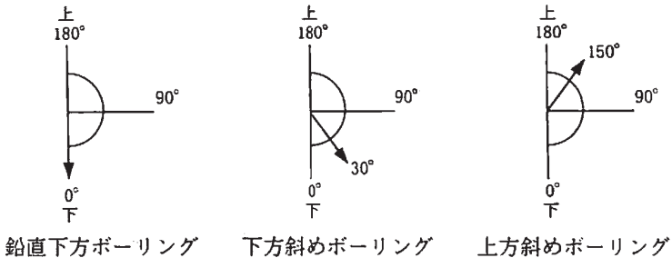
図2. 2 ボーリングの角度の表示例
