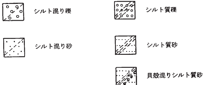
図3. 6 第1分類と第2分類の組合せの例
