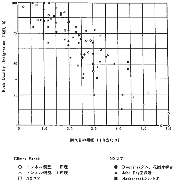
図 5. 2 RQDと割れ目の頻度との関係 15)
