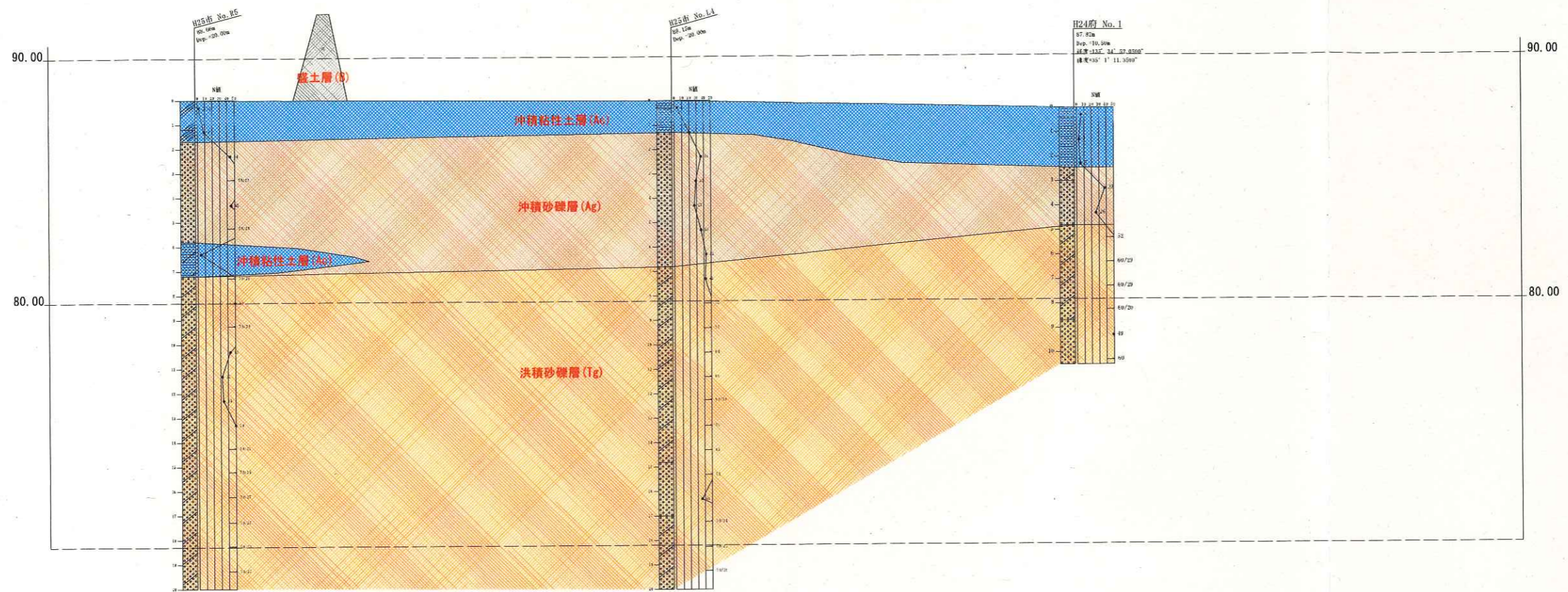
地質想定断面図（西—東方向） H=1:2000 V=1:200
