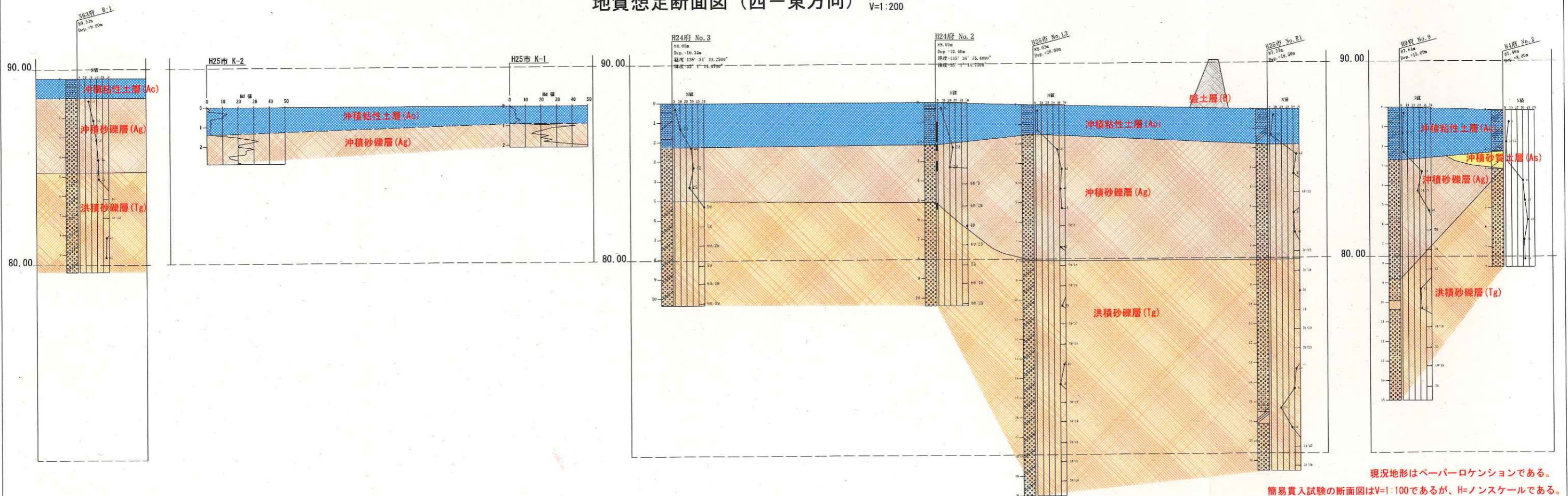
地質想定断面図（西—東方向） H=1:2000 V=1:200
