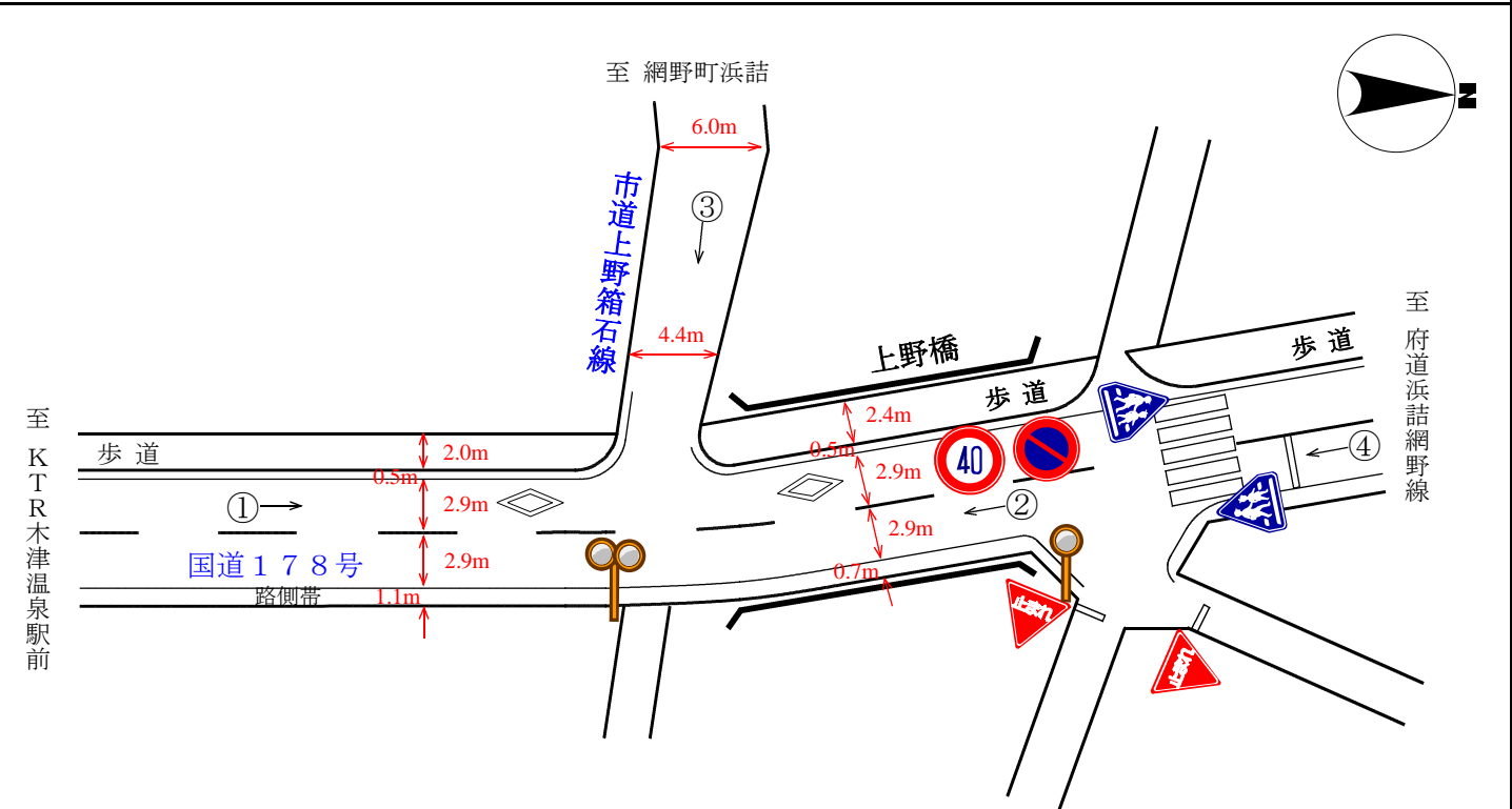
交差点図面
