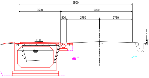
標準横断図
